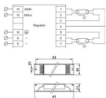
Scheda tecnica Philips HF-Ri TD 2 28-54 TL5 E+ 195-240V
